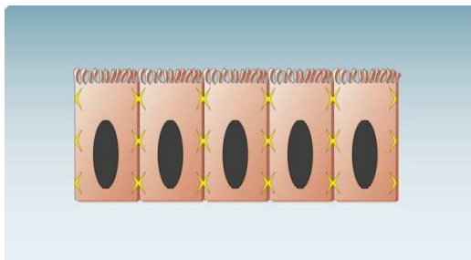
Abb. Abb. 2: Tight Junctions zwischen Enterozyten, schematische Darstellung
