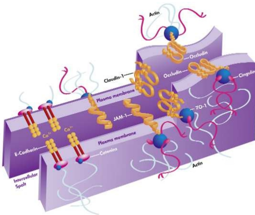
Abb. 1: Tight Junction, schematische Darstellung
